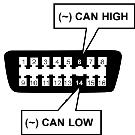
④ OBD-II connector Connecteur OBD-II
